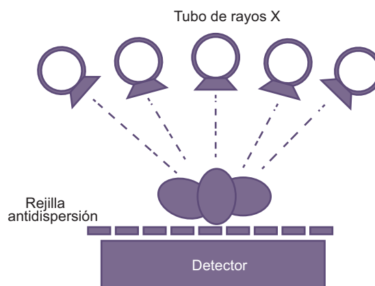
Figura 1-2 Esquema de una tomosíntesis digital. Arriba, el tubo de rayos X deslizándose de forma paralela al paciente irradiado. El panel detector plano se encuentra debajo de la rejilla. La técnica permite que el tubo de rayos X se incline en varios ángulos para que pueda seguir una trayectoria definida y paralela al detector mientras se adquieren las imágenes.
